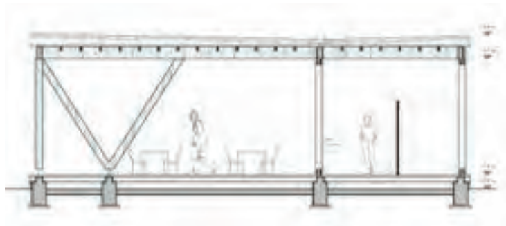
sezione trasversale
